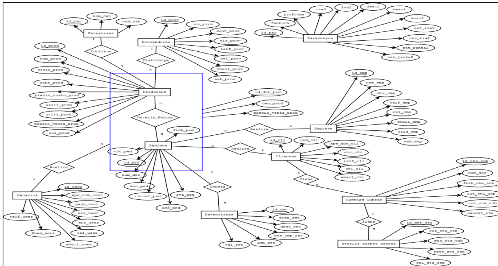
Figura N° 3. Diagrama Entidad Relación (Sif).
