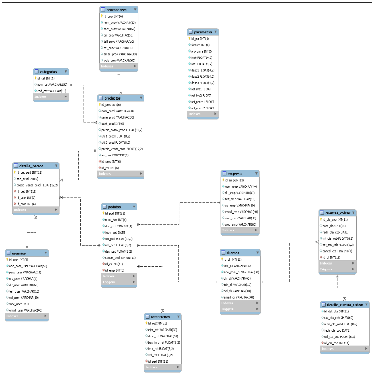
Figur N°4. Diagrama de la Base de Datos (Sif).
