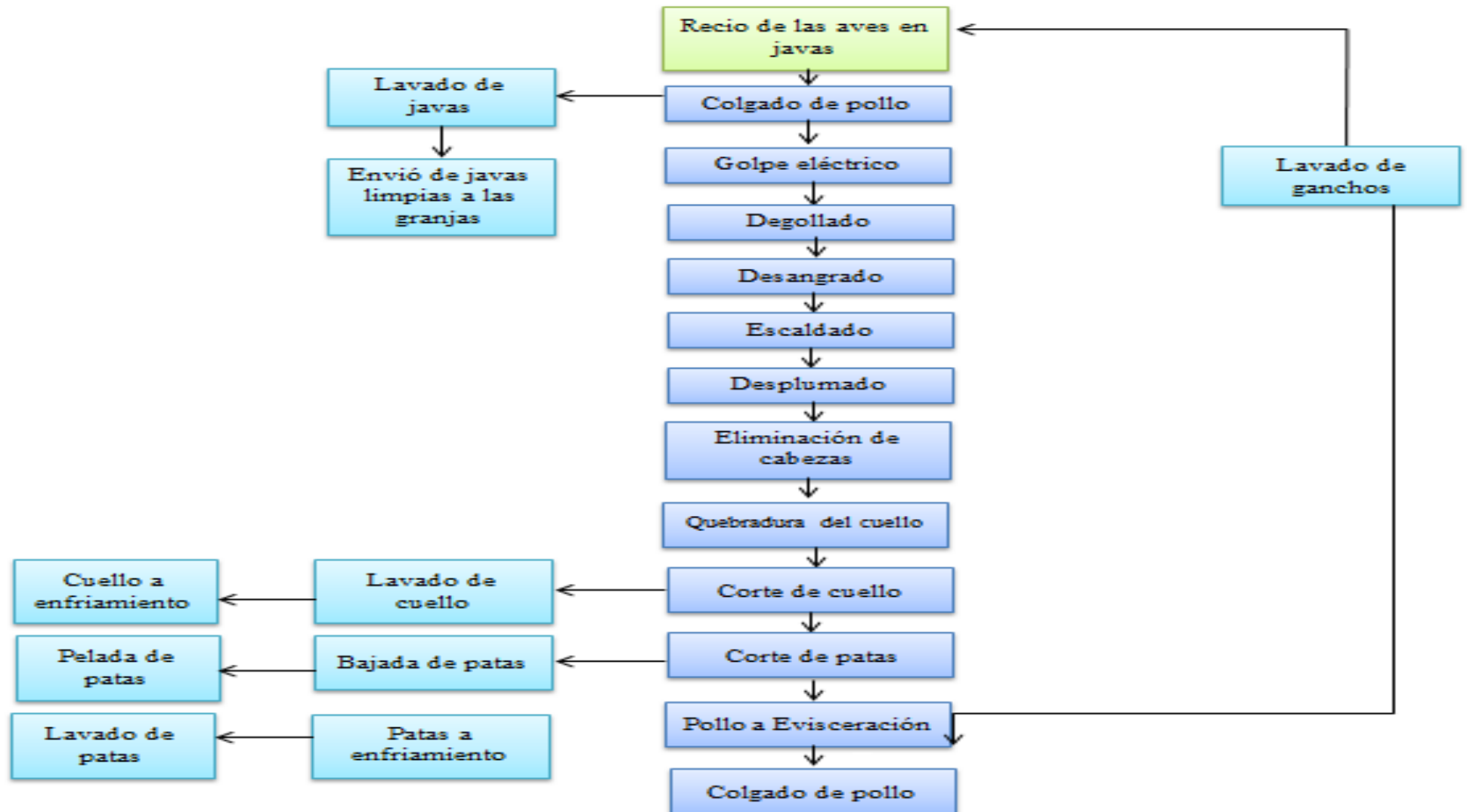
Flujograma N° 2: Diagrama de Flujo de proceso de Pollo
